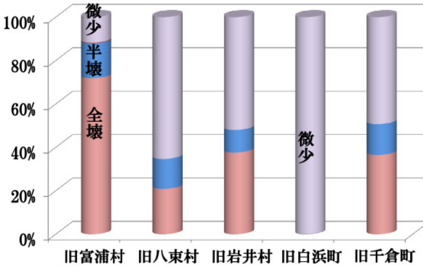
図1. 関東大震災時の家屋の被害状況
